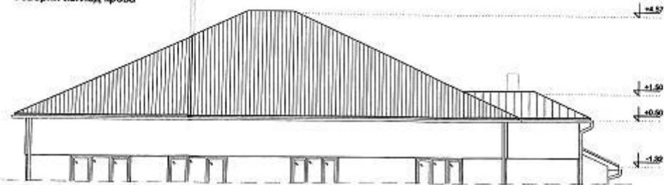
Северни изглед на крова
